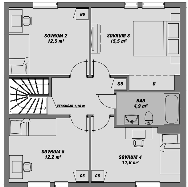
OVANVÅNING BOA - 69,3 m 2
